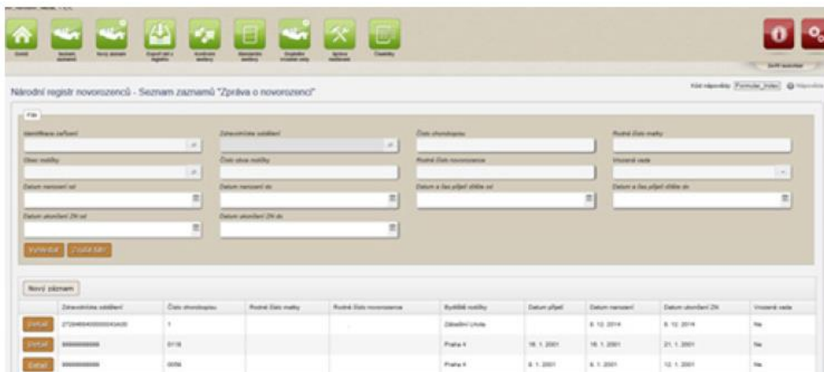
Obrázek 21 – Vyhledávání záznamů
