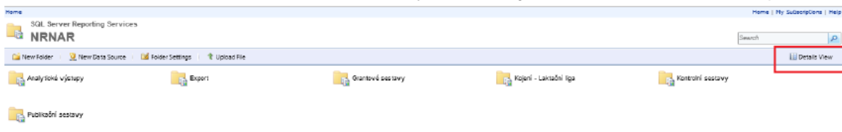
Obrázek 25 – Details View
